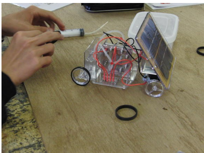
自動車・燃料電池自動車模型実験
